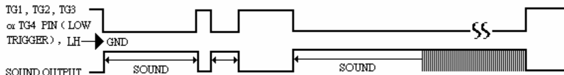
TRIGGER MODE : LEVEL HOLD
